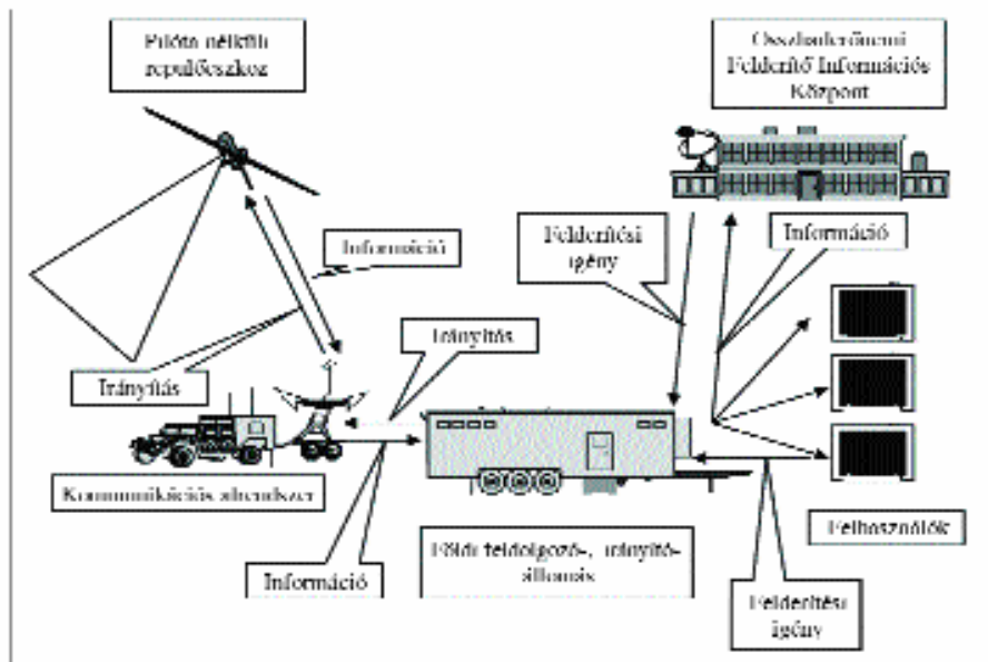
1. ábra A pilóta nélküli repülőeszköz (rendszer) működési vázlatja
